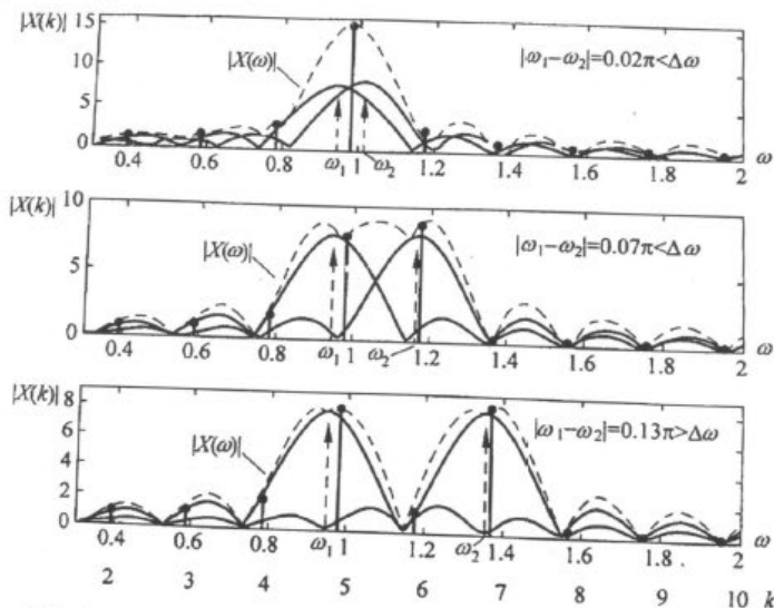
图 3-25 连续频谱和 16 点 DFT 的幅度(局部图形), \Delta\omega = 0.125\pi
