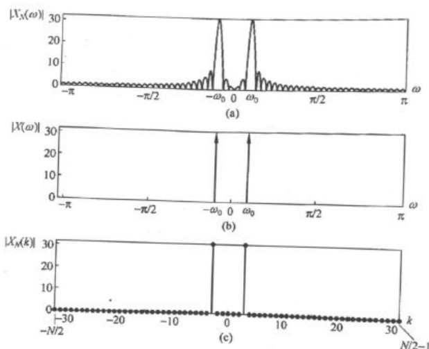
图 3-19 长为 N=64 的正弦序列 ( M=3 ) 的 DTFT 和 DFT 的幅度
