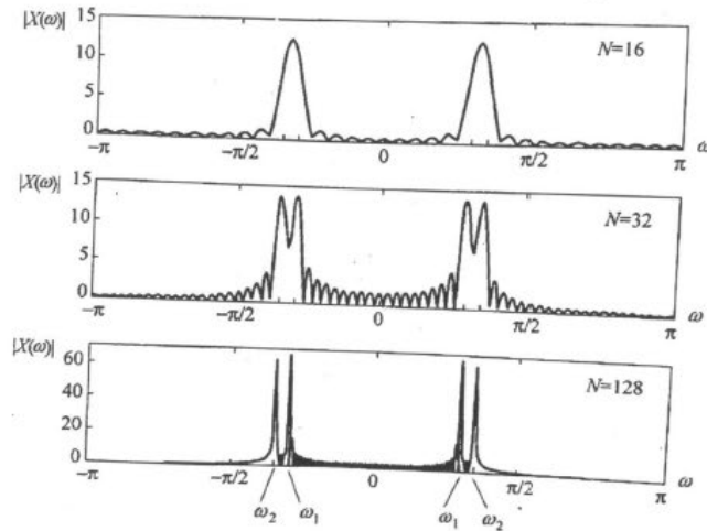
图 3-20 说明取样点数对频率分辨率影响的例子
